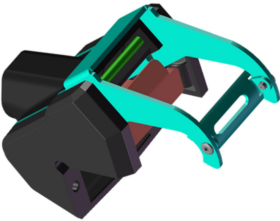
设计1立体图
