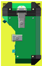
设计2左视图
